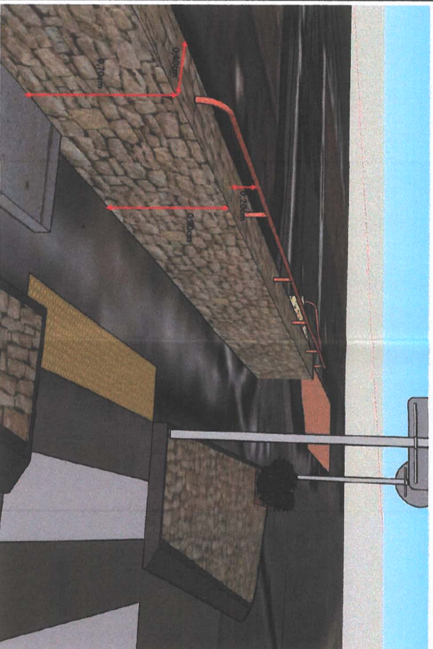
CROQUIS DE PRINCIPLE MISE EN PLACE D'UNE LISSE SUR LE PARAPET
